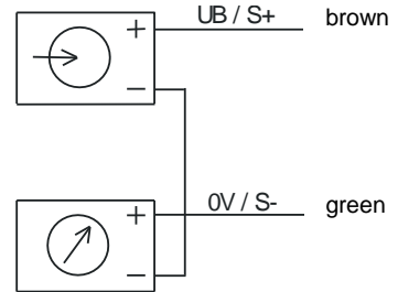
cable outlet
